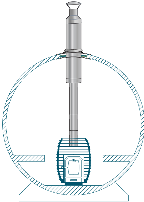
KAMINSET FÜR FASSAUNEN
