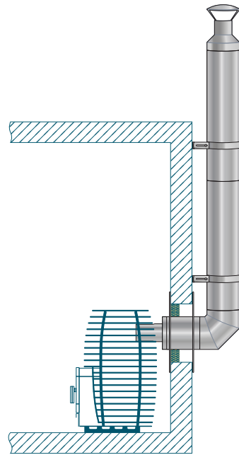
KAMINSET WANDDURCH- FÜHRUNG ANSCHLUSS RÜCKSEITE
