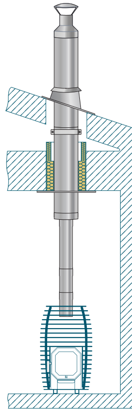
KAMINSET MIT DACHDURCHFÜHRUNG
