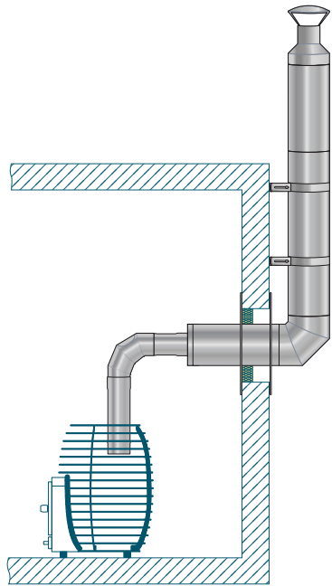
KAMINSET WANDDURCH- FÜHRUNG ANSCHLUSS OBERSEITE
